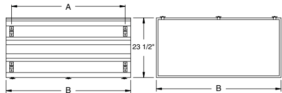
4 FT LUMINAIRE
