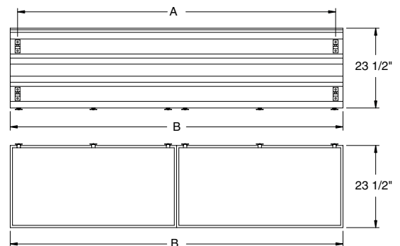
8 FT LUMINAIRE
